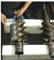
Đo đường kính ngoài của trục vít
